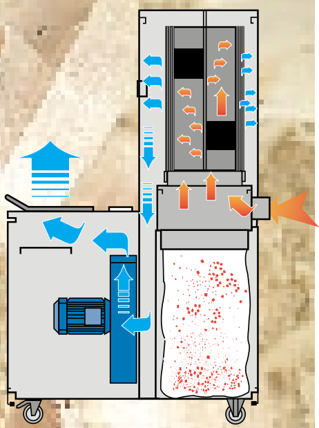
EUROFILTER 100-140-160
